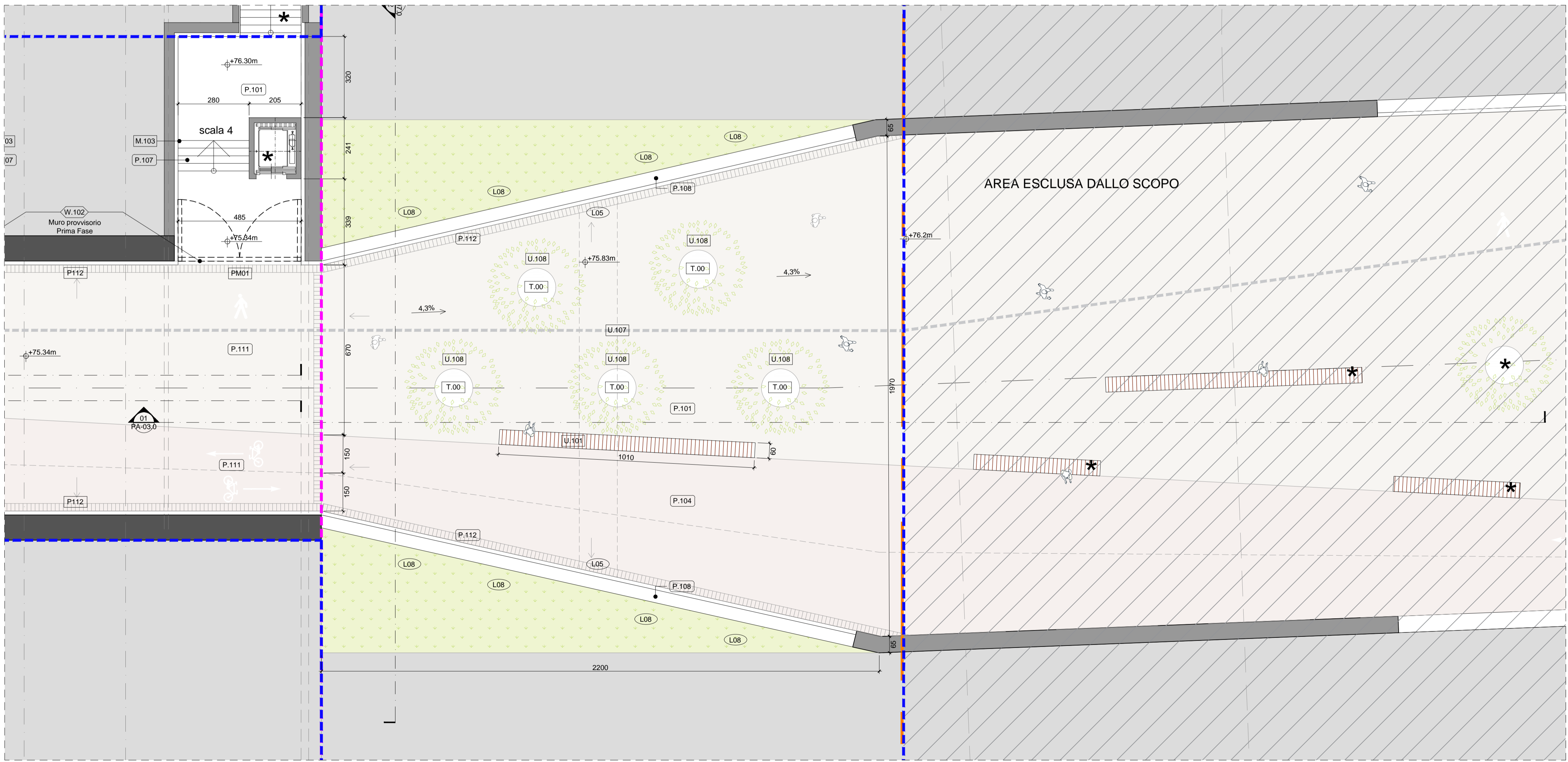
02 PIANTA QUOTA SOTTOPASSO INGRESSO LATO NECCHI 1:100
