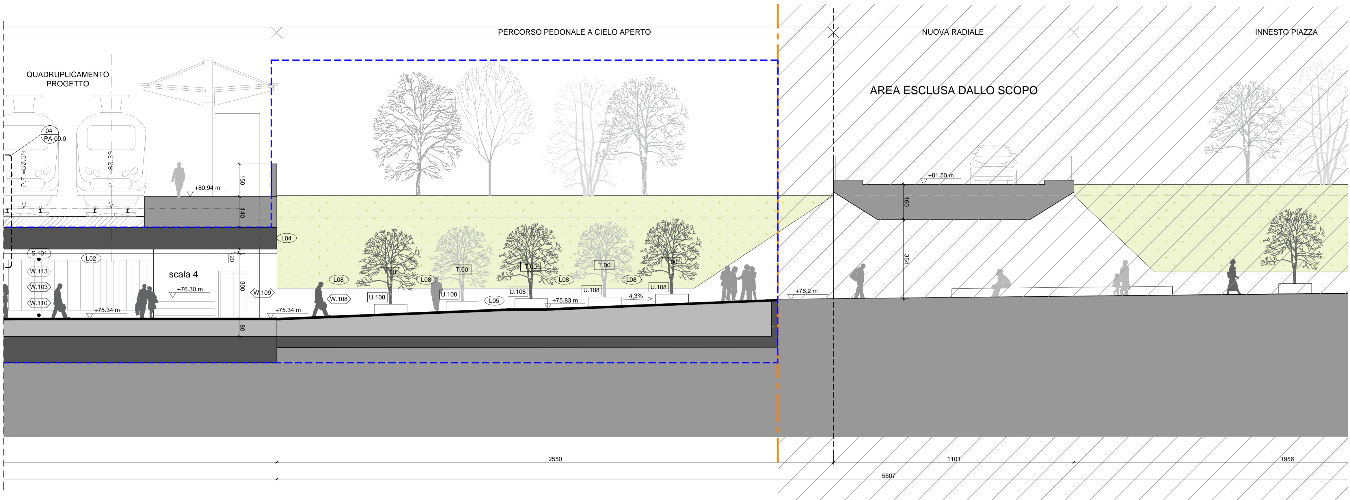
01 SEZIONE AA' - SOTTOPASSO INGRESSO LATO NECCHI 1:100
