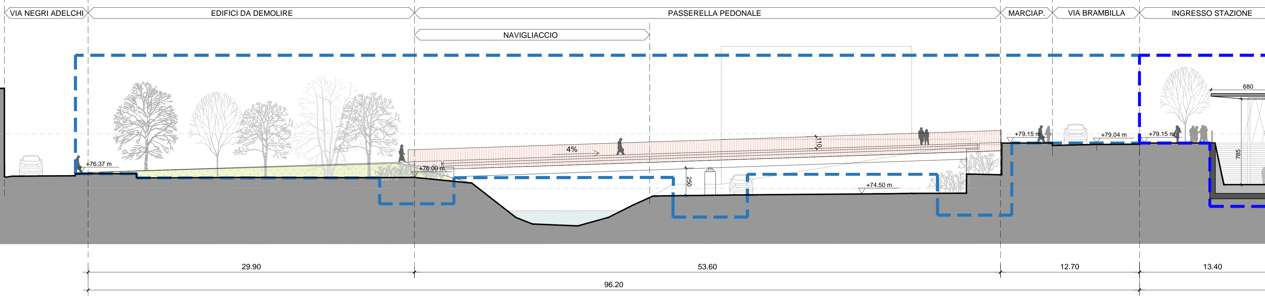
01 PROSPETTO PASSERELLA CICLOPEDONALE 1:200
