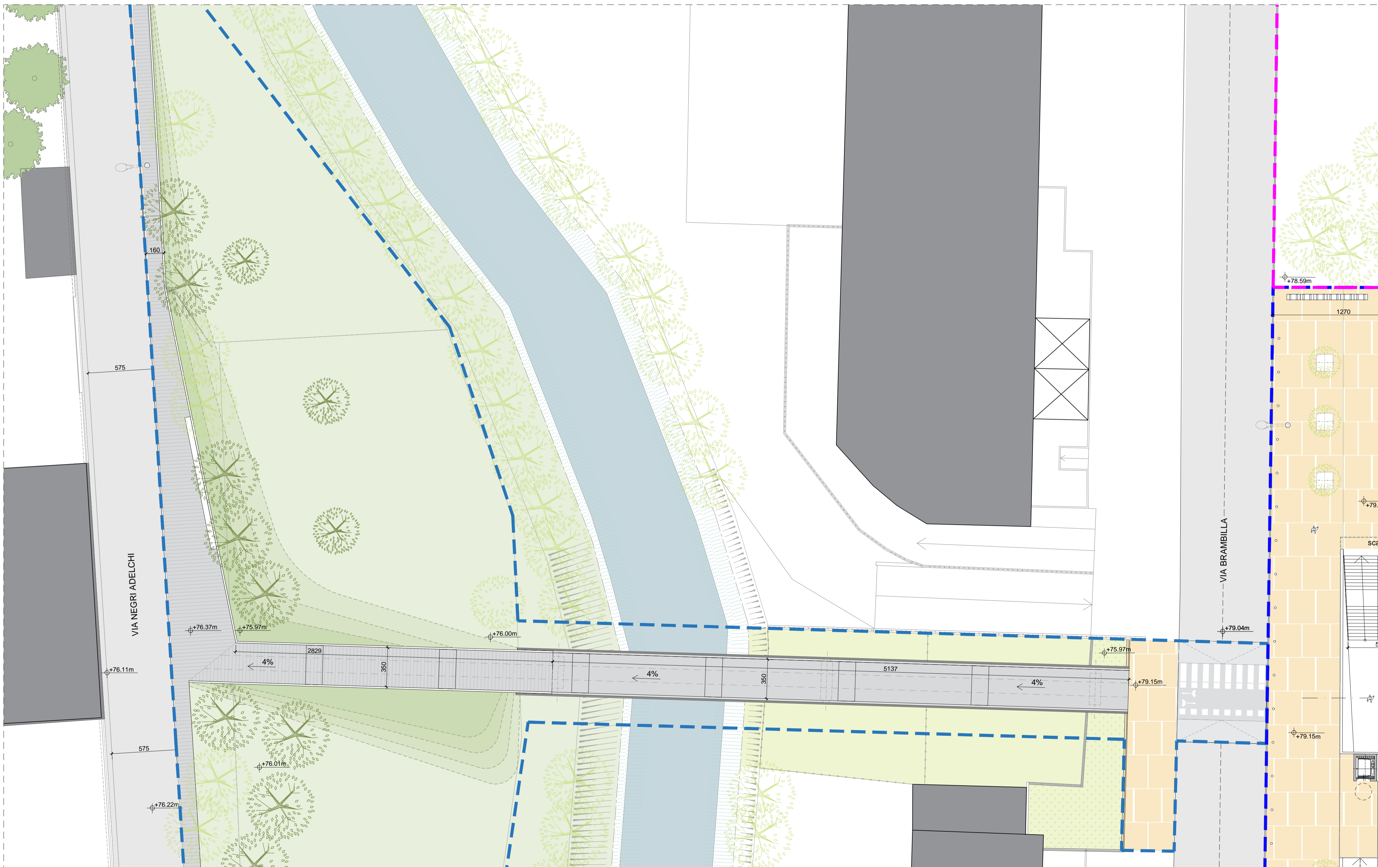
02 PIANTA PASSERELLA CICLOPEDONALE 1:200
