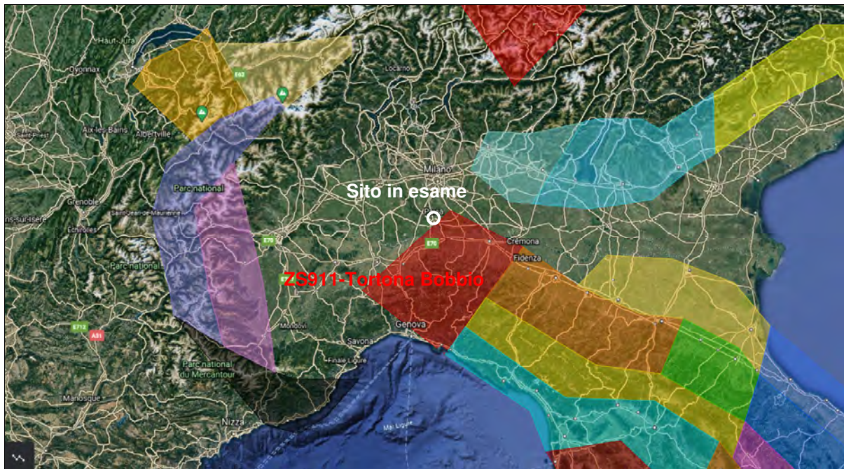
Figura 19: Zonazione Sismogenetica ZS9 (stralcio da https://earth.google.com/web )
