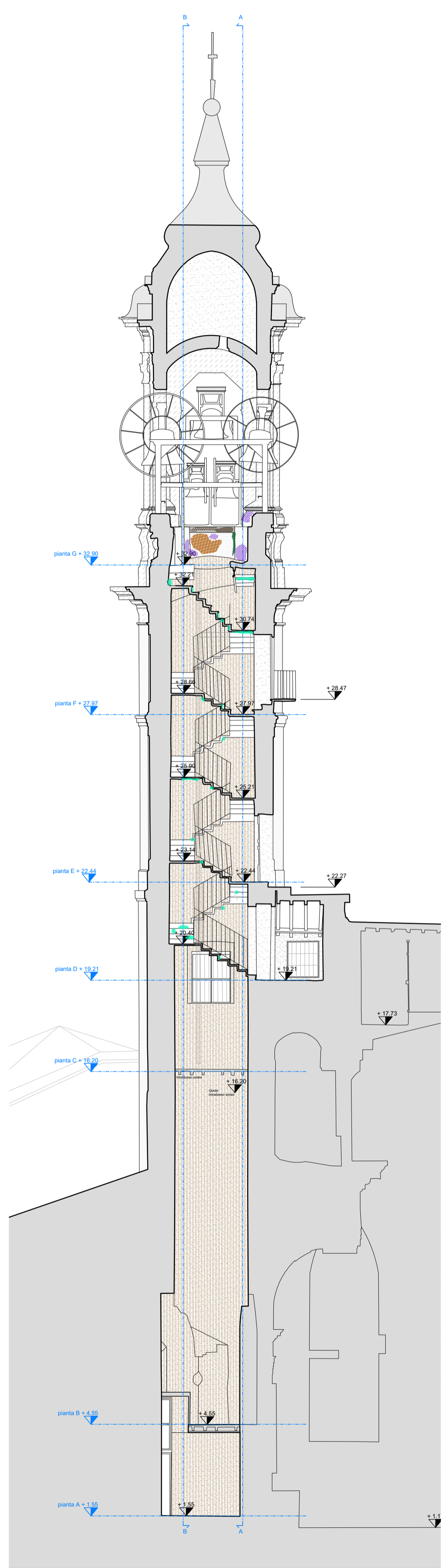
03 STATO DI FATTO - SEZIONE C-C' 1:100
