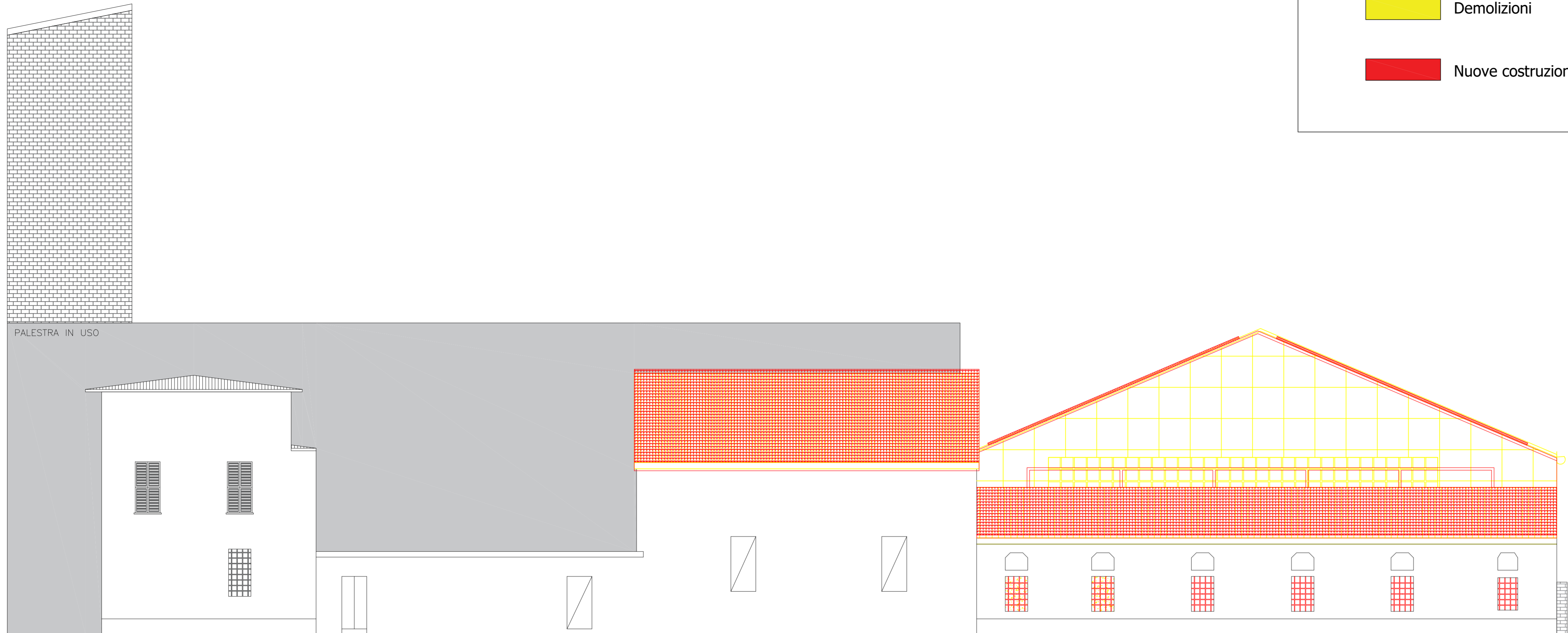
Prospetto Sud Scala 1:100
