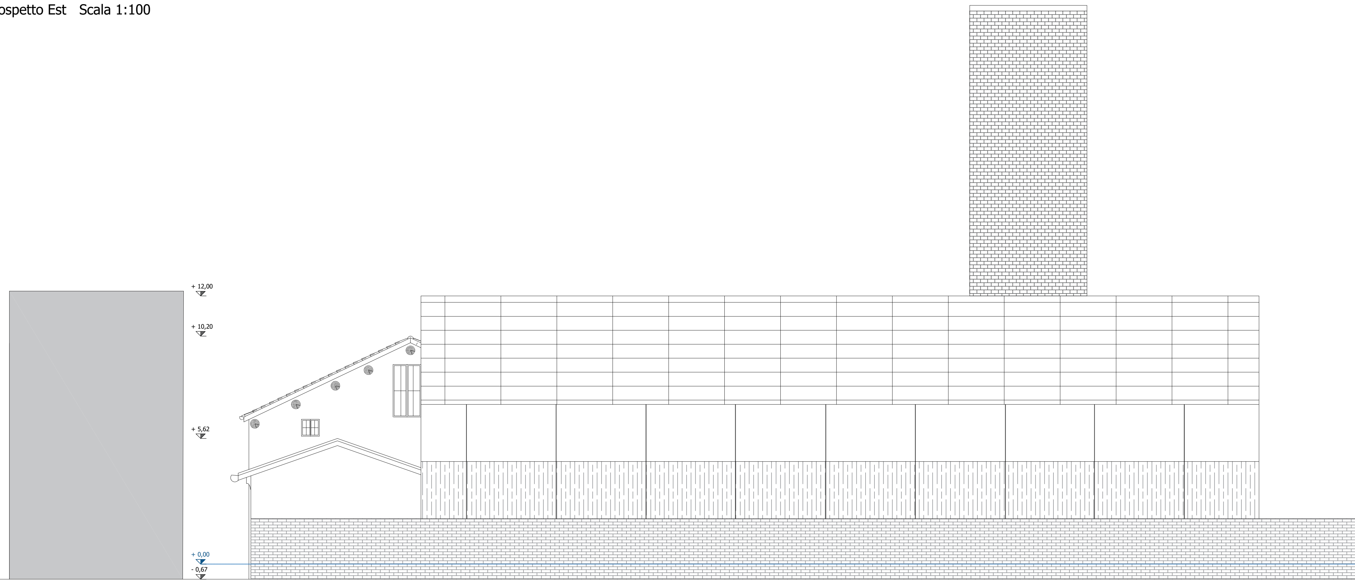
Prospetto Est Scala 1:100
