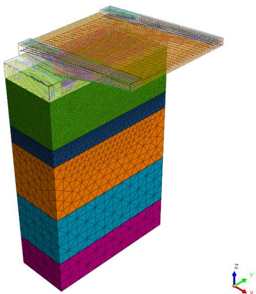
Vista 3d – Struttura e terreno
