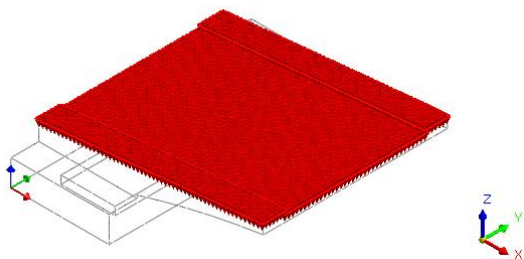
Carico distribuito – Q neve
