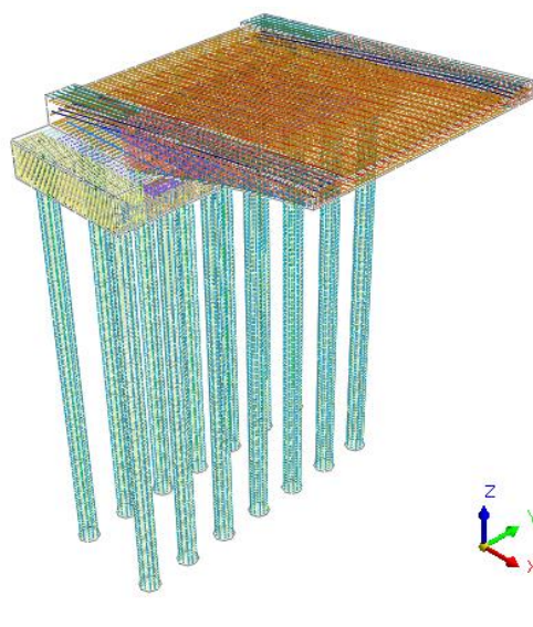
Vista 3d – Struttura
