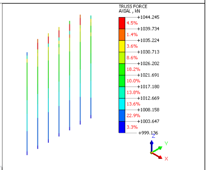
Stato di sforzo assiale - cavi di post tensione
