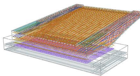
Vista 3d laterale – Armatura impalcato e piastra di fondazione
