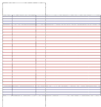
Vista in pianta – Cavi di post tensione impalcato
