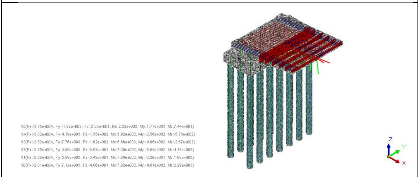
Section Cut - Impalcato
