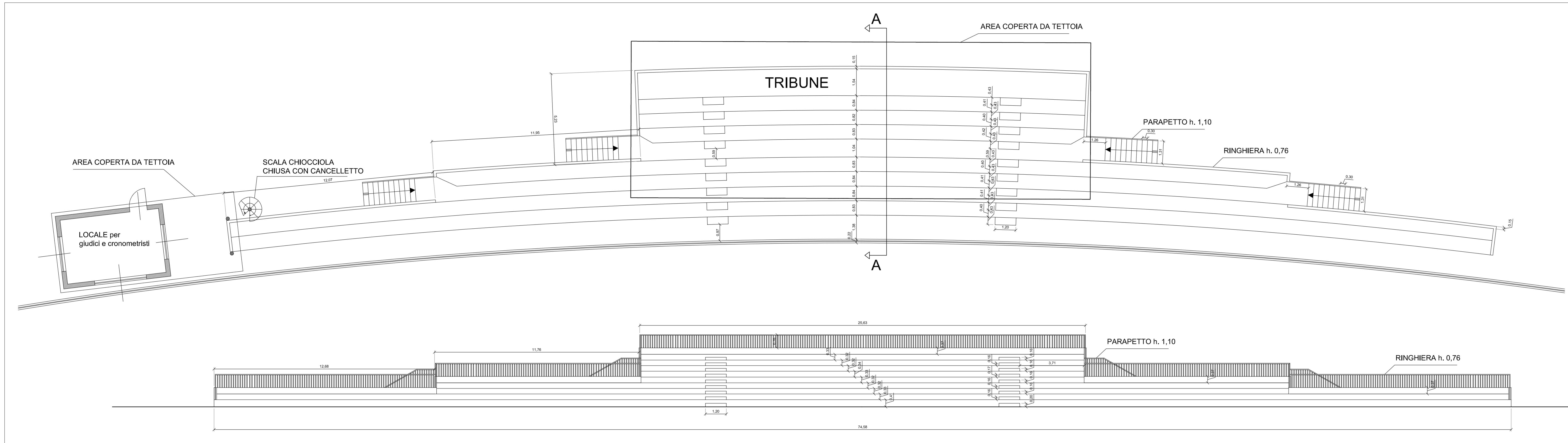
STATO DI PROGETTO - PIANTE E PROSPETTO FRONTALE - SCALA 1:100
