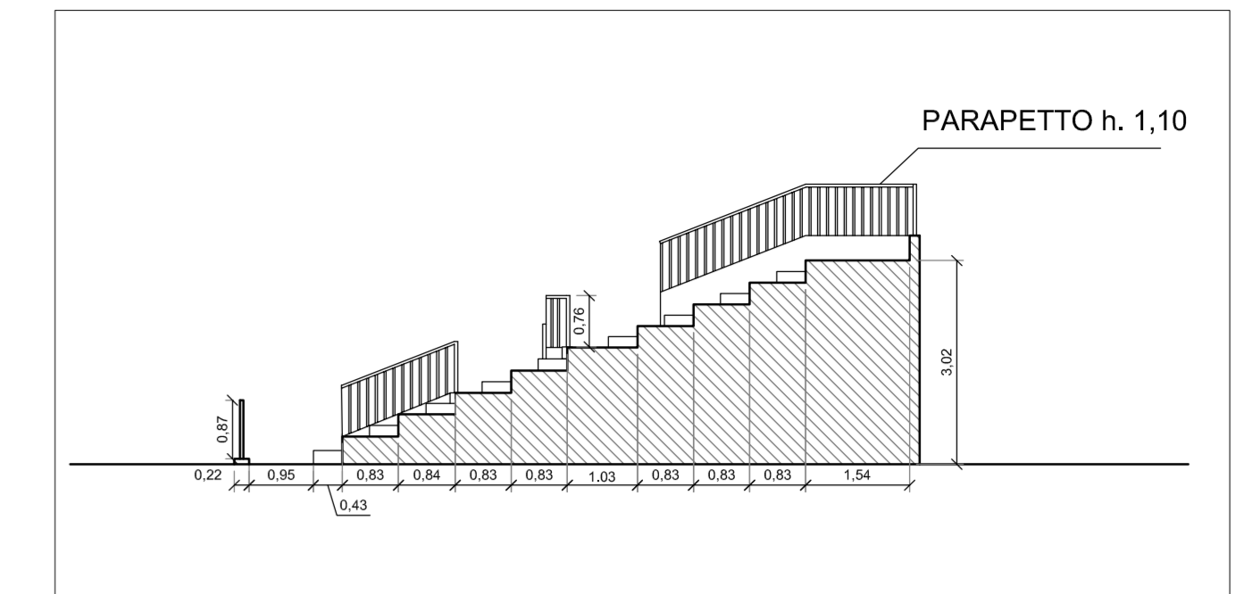
STATO DI PROGETTO - SEZIONE AA - SCALA 1:100
