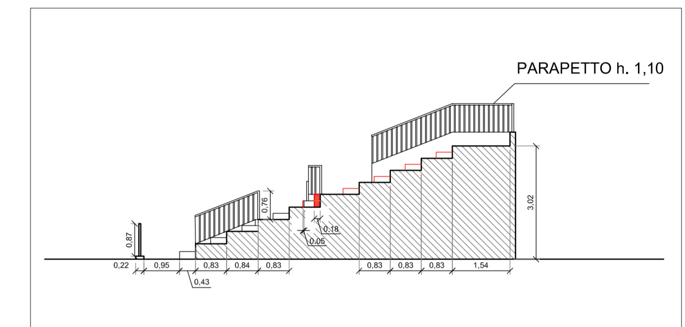
STATO DI CONFRONTO - SEZIONE AA - SCALA 1:100
