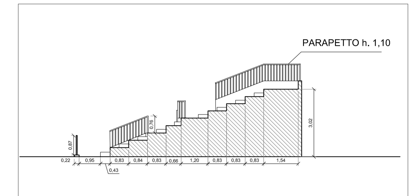
STATO DI CONFRONTO - SEZIONE AA - SCALA 1:100
