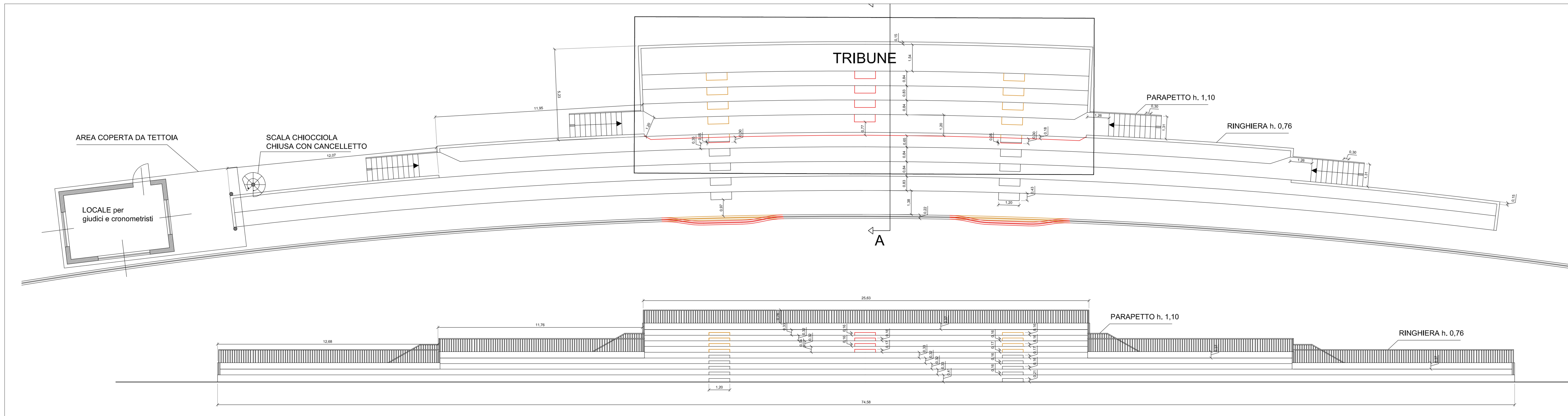
STATO DI CONFRONTO - PIANTE E PROSPETTO FRONTALE - SCALA 1:100
