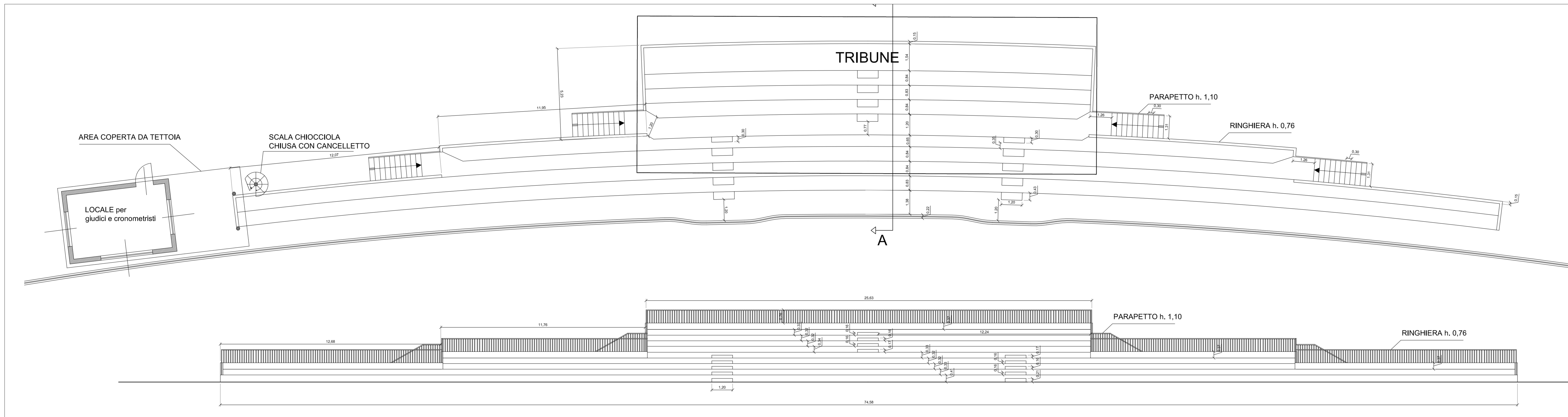
STATO DI PROGETTO - PIANTE E PROSPETTO FRONTALE - SCALA 1:100
