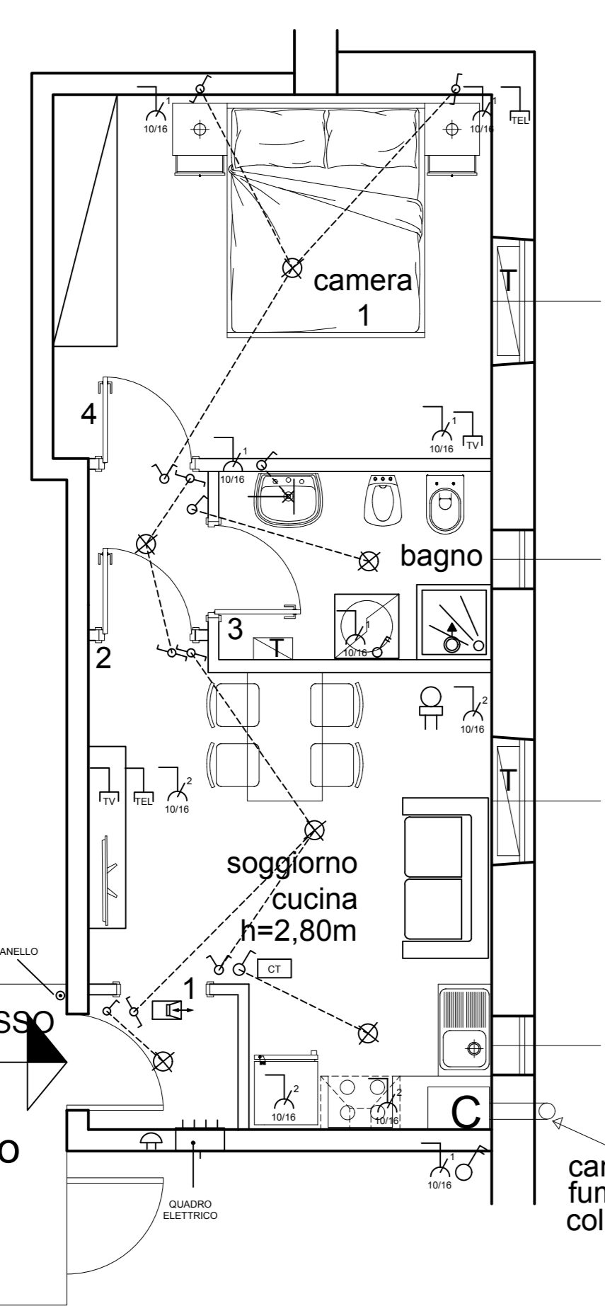
Crosione (16) GRADINARU, piano rialzato Catasto: Foglio B 16, mapp. 1390 sub.19 SCALA 1:50 (IMPIANTI STATO DI PROGETTO)
