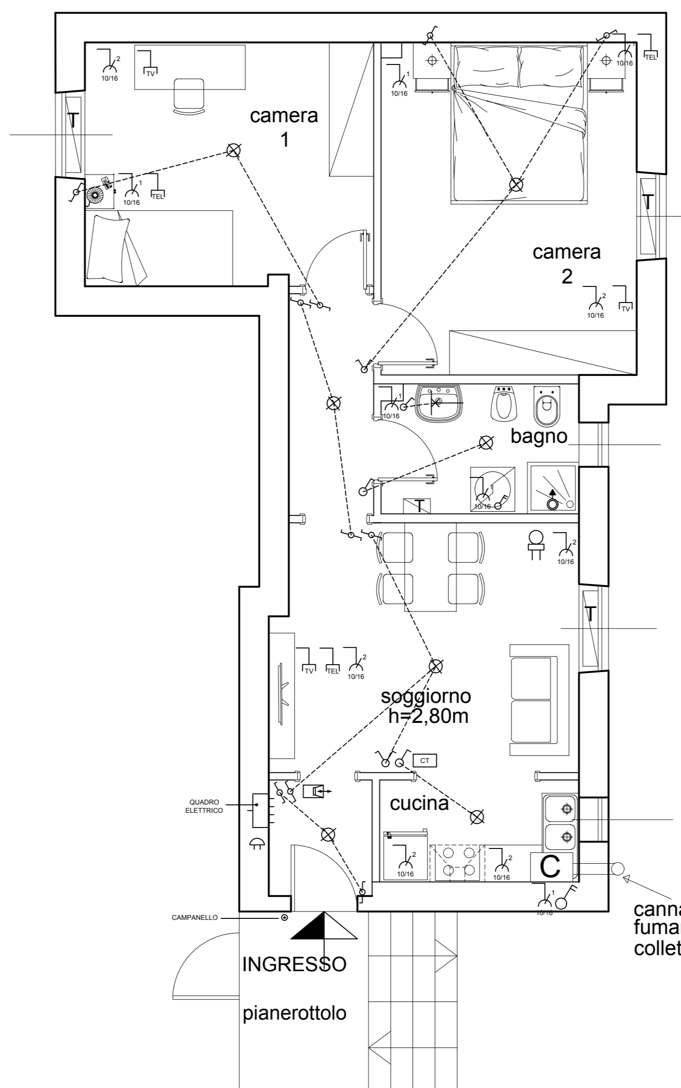
Crosione (18) MORANDI, 3° piano Catasto: Foglio B 16, mapp. 1391 sub 16 SCALA 1:50 (IMPIANTI STATO DI PROGETTO)
