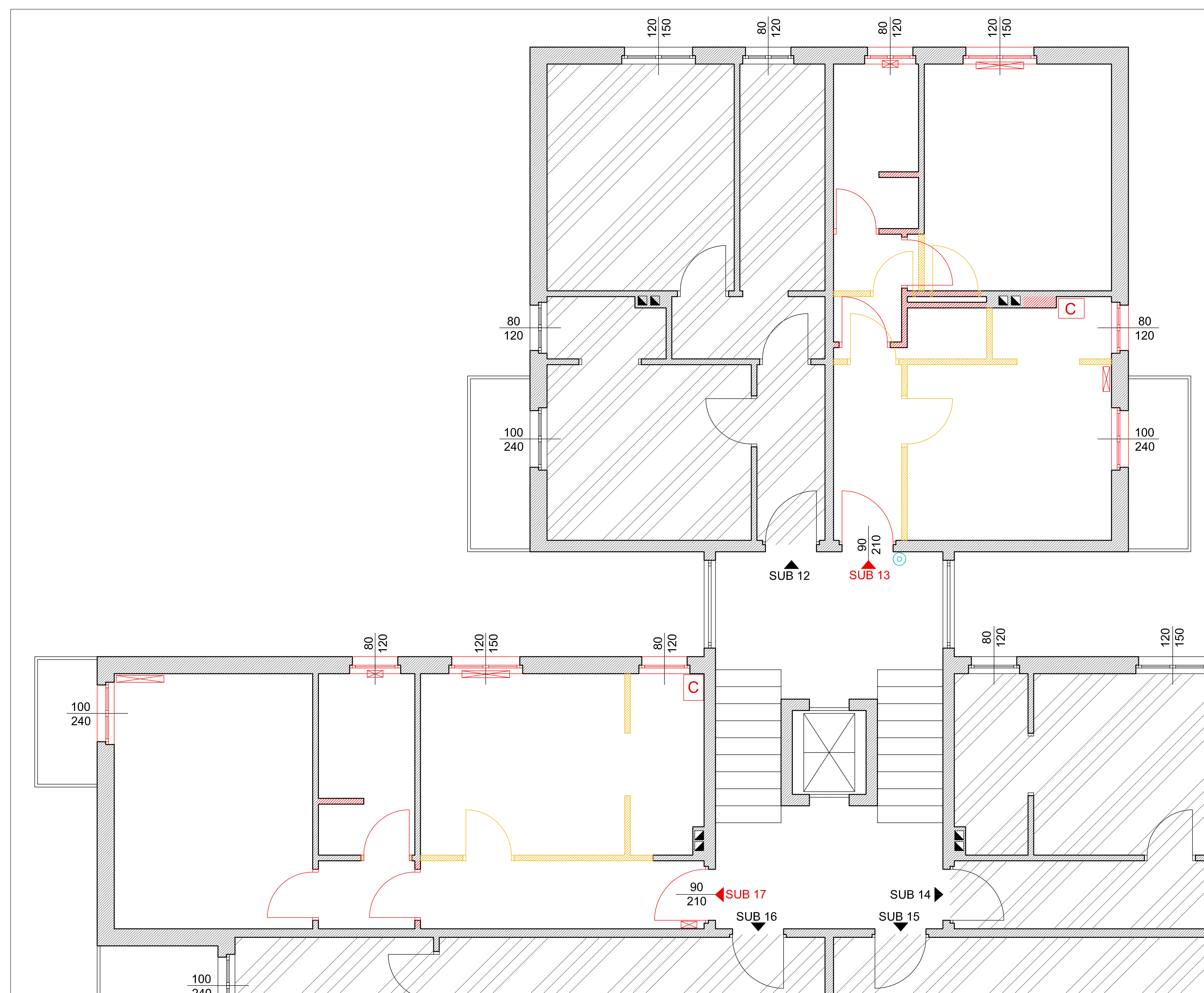
STATO DI CONFRONTO - PIANO SECONDO - SCALA 1:50
