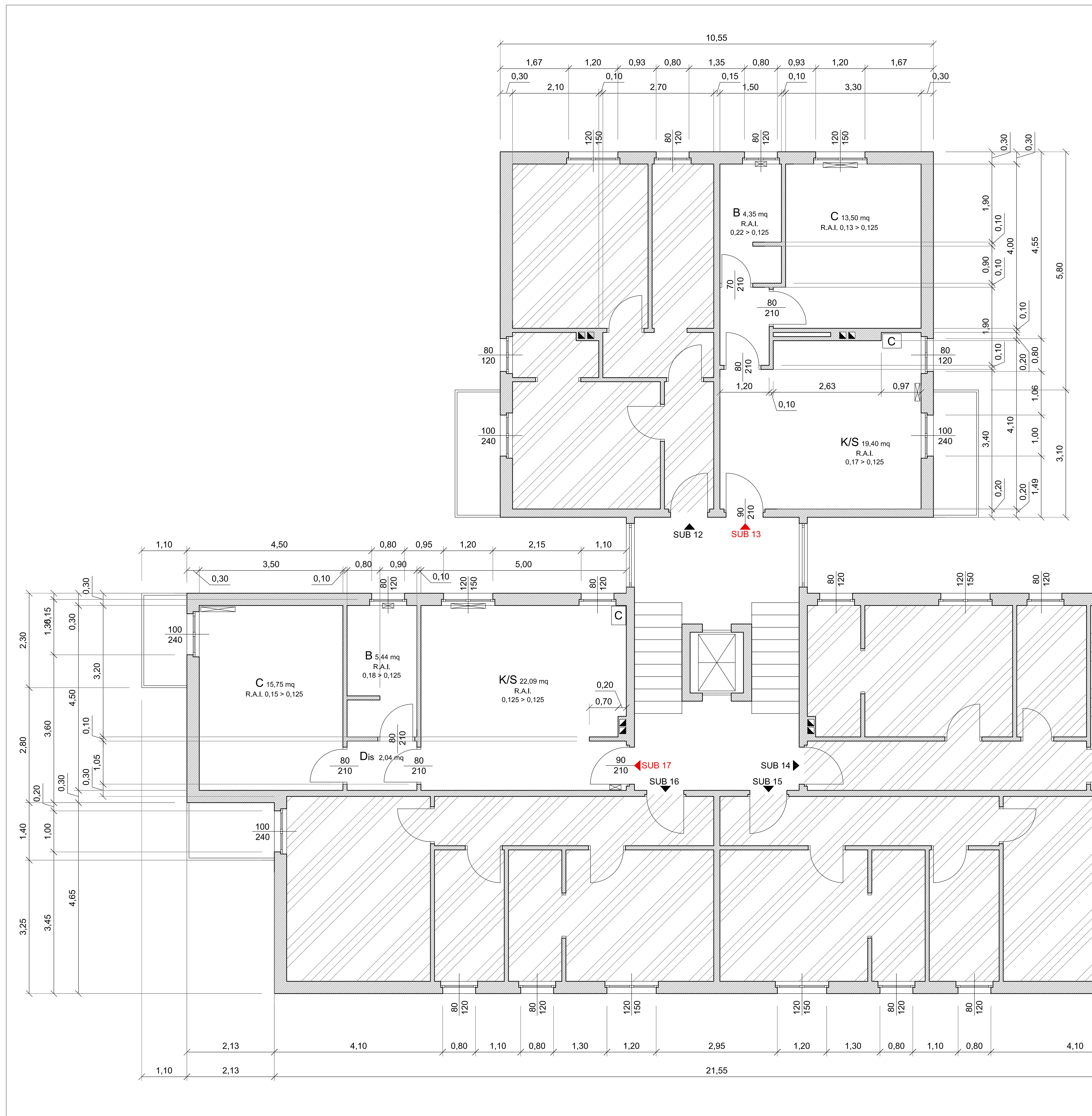
PIANTA QUOTATA - PIANO TERZO - SCALA 1:50
