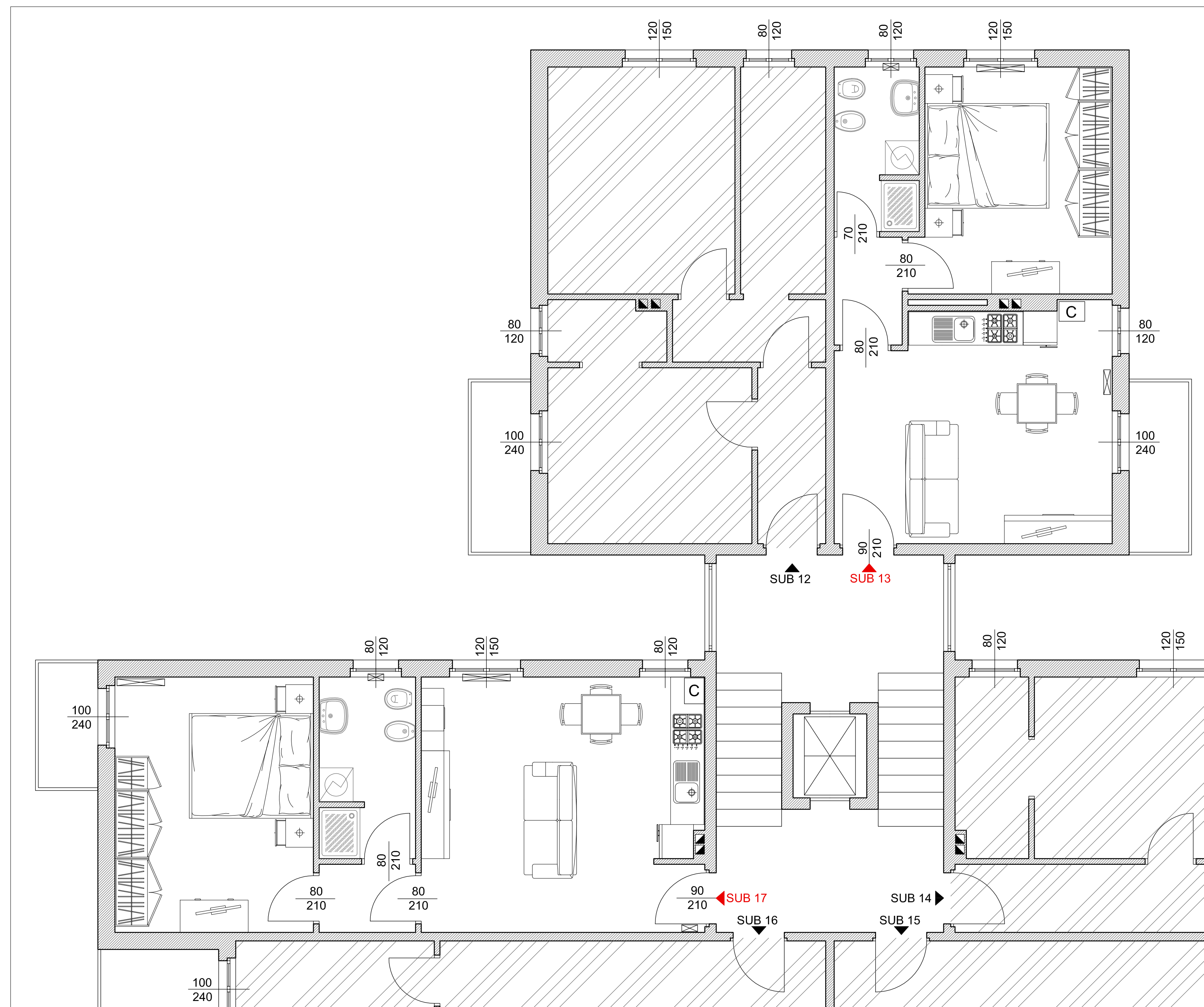
STATO DI CONFRONTO - PIANO SECONDO - SCALA 1:50
