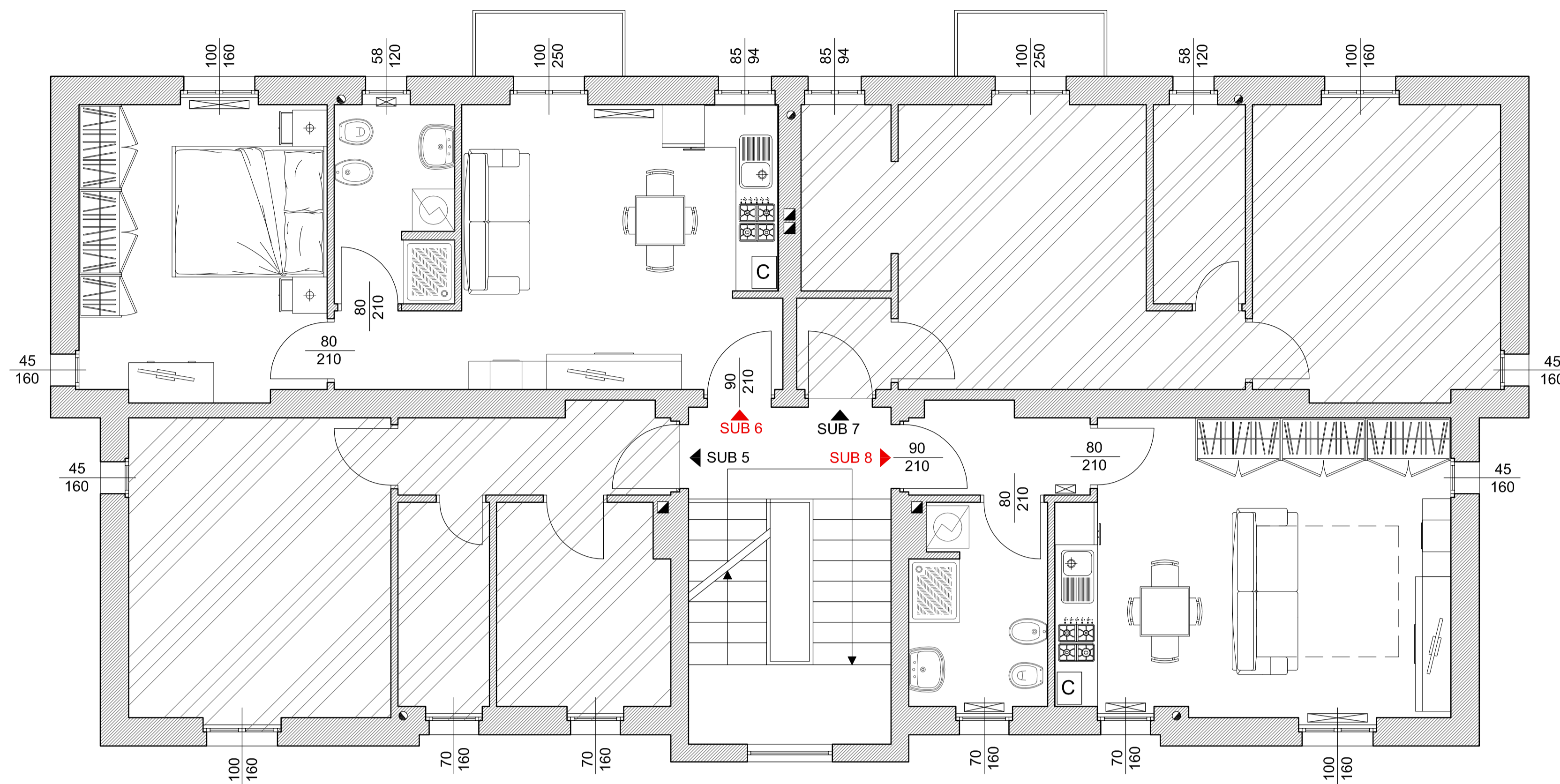
PIANTA QUOTATA - PIANO PRIMO - SCALA 1:50
