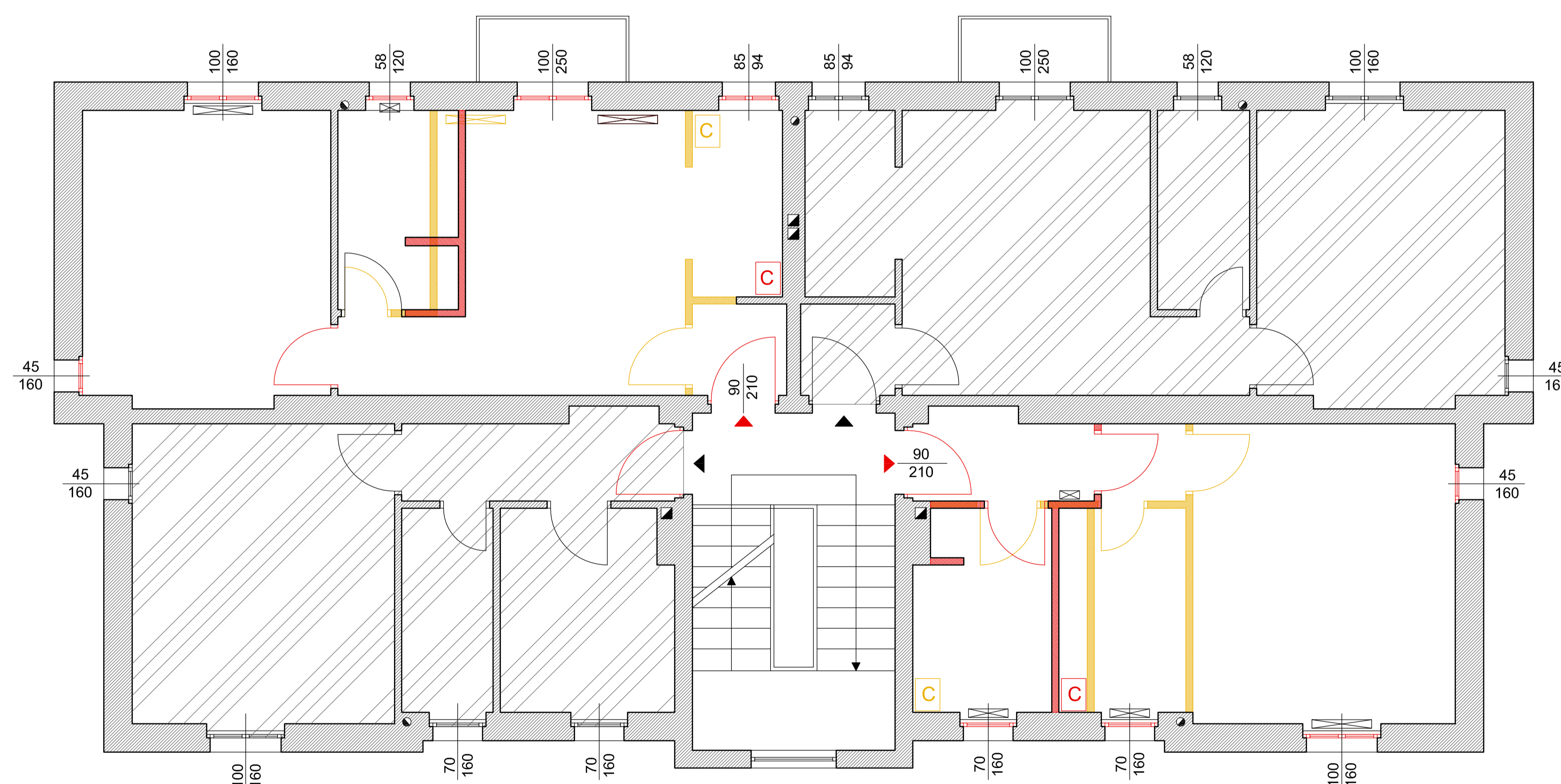
STATO DI CONFRONTO - PIANO PRIMO - SCALA 1:50
