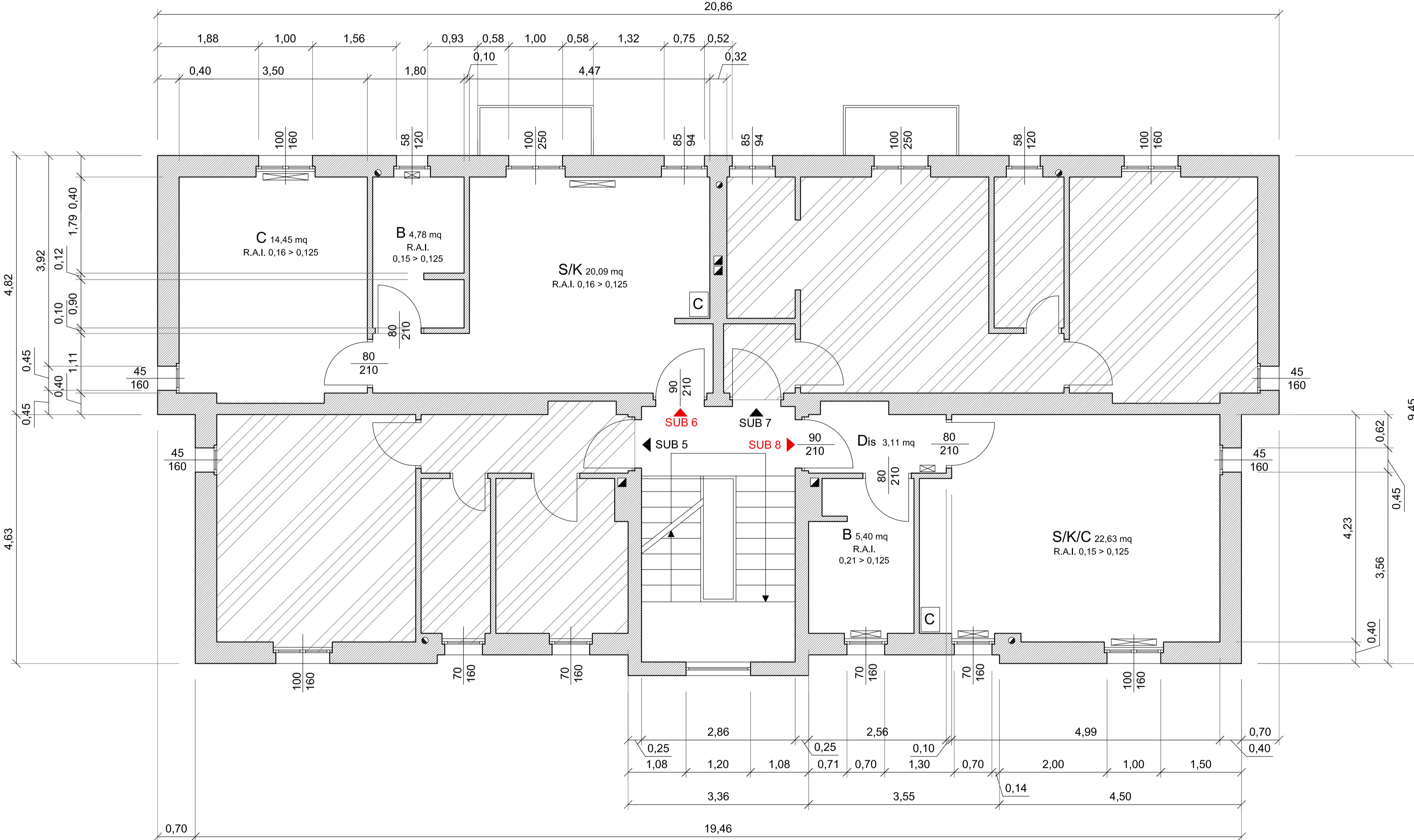
STATO DI CONFRONTO - PIANO PRIMO - SCALA 1:50
