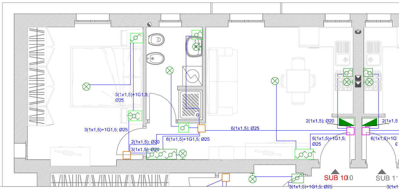
PIANTA IMPIANTO LUCI - VIA VIVAI 3/A, PAVIA - PIANO SECONDO, SUB 10 - SCALA 1:50
