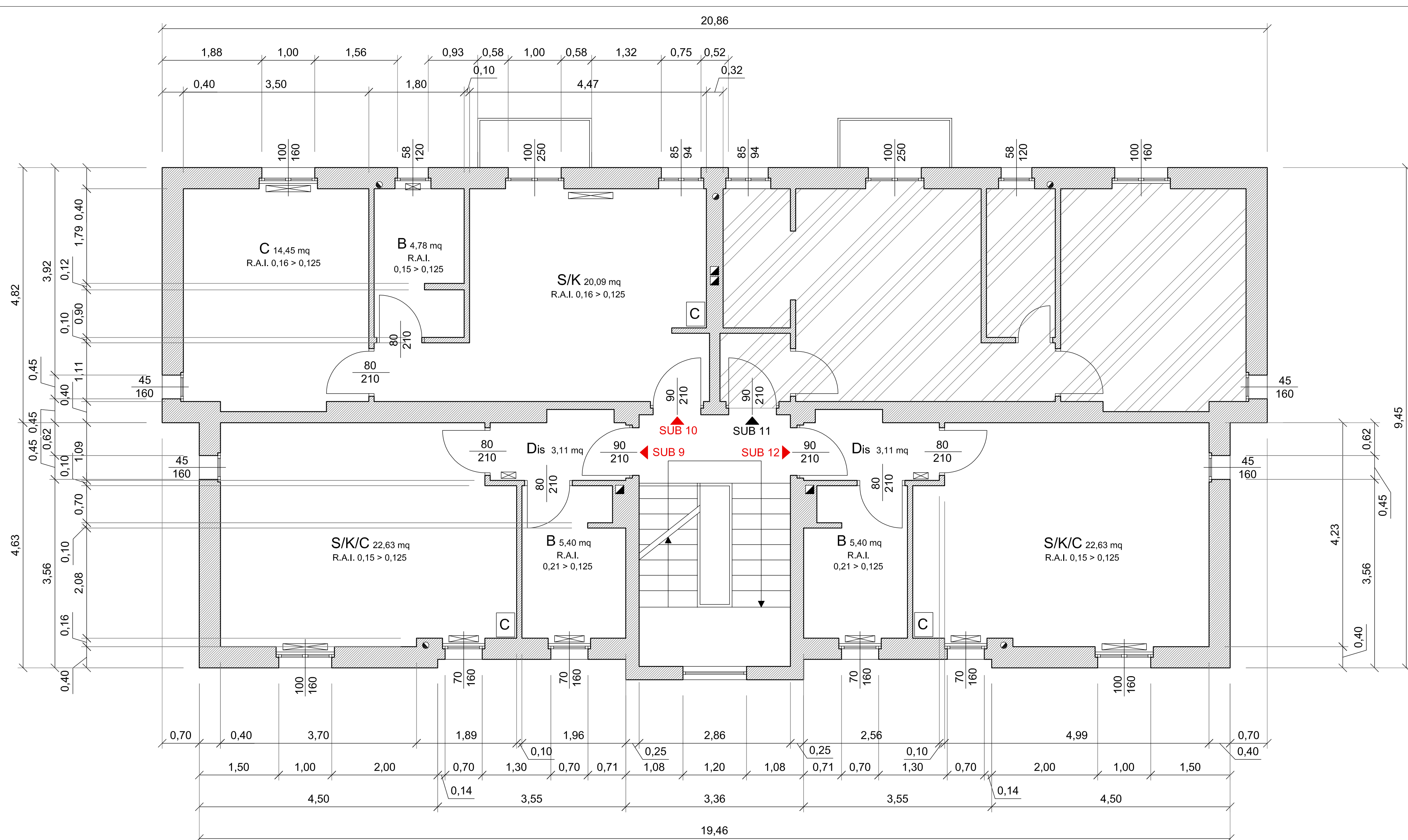
PIANTA QUOTATA - PIANO SECONDO - SCALA 1:50
