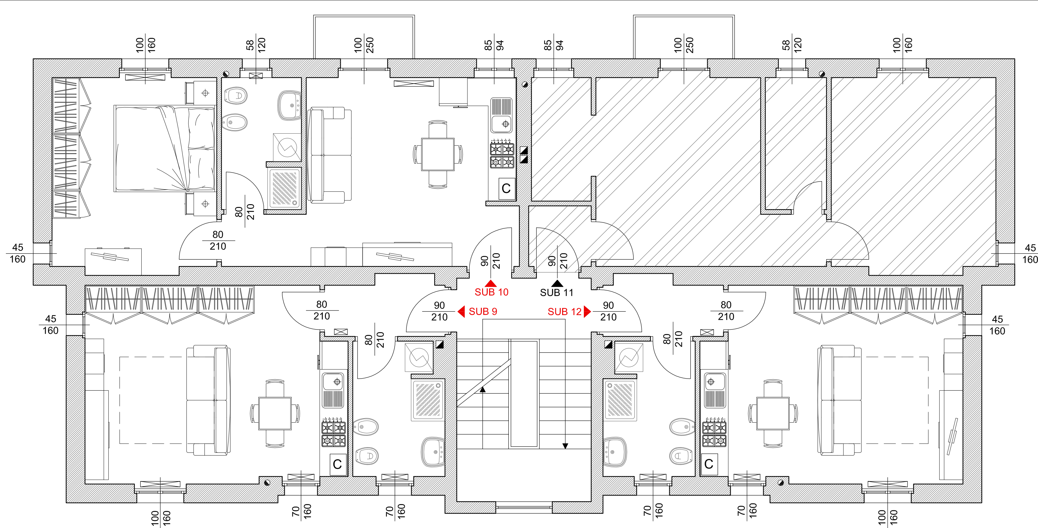
PIANTA ARREDATA - PIANO SECONDO - SCALA 1:50
