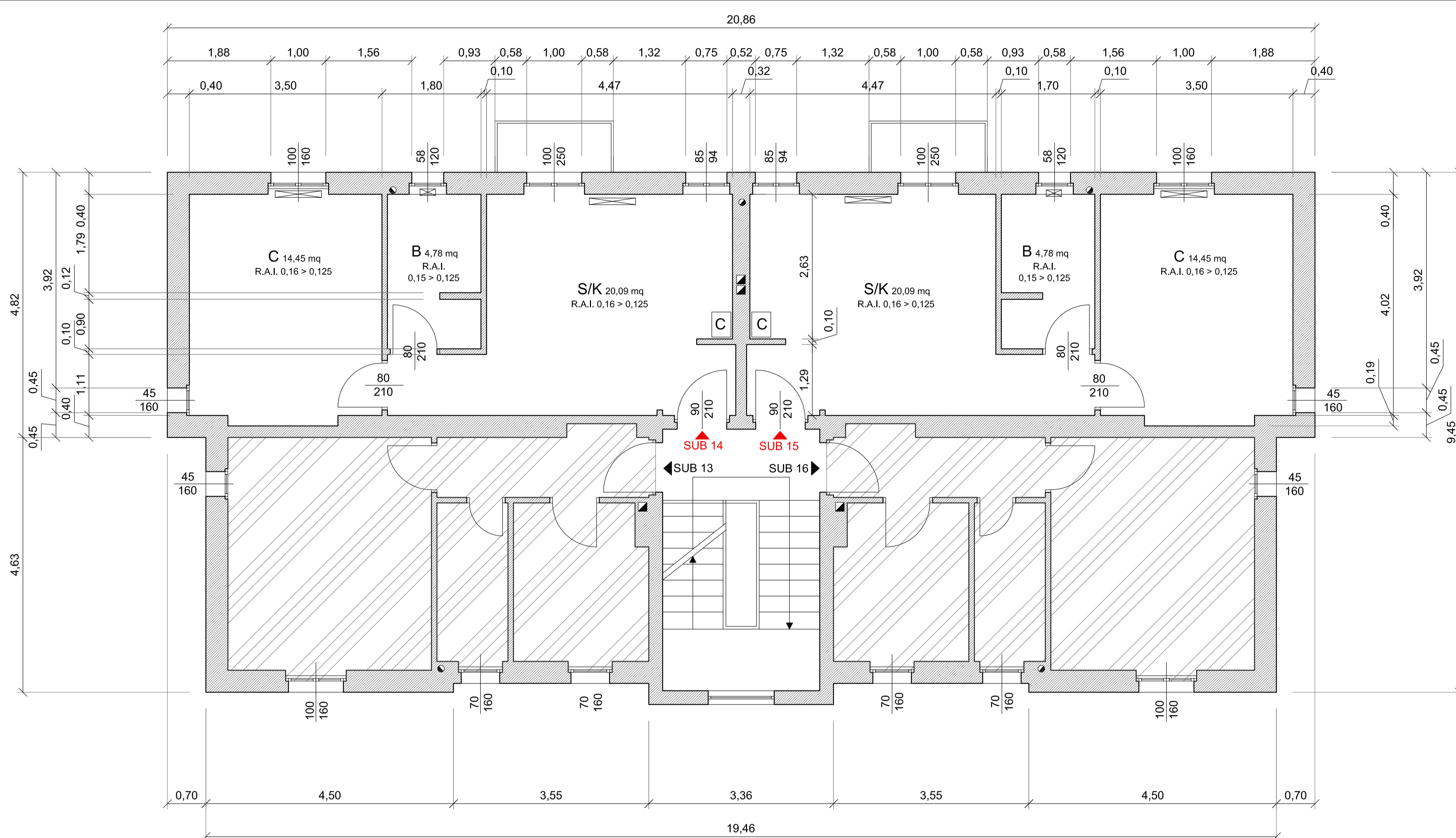
PIANTA QUOTATA - PIANO TERZO - SCALA 1:50
