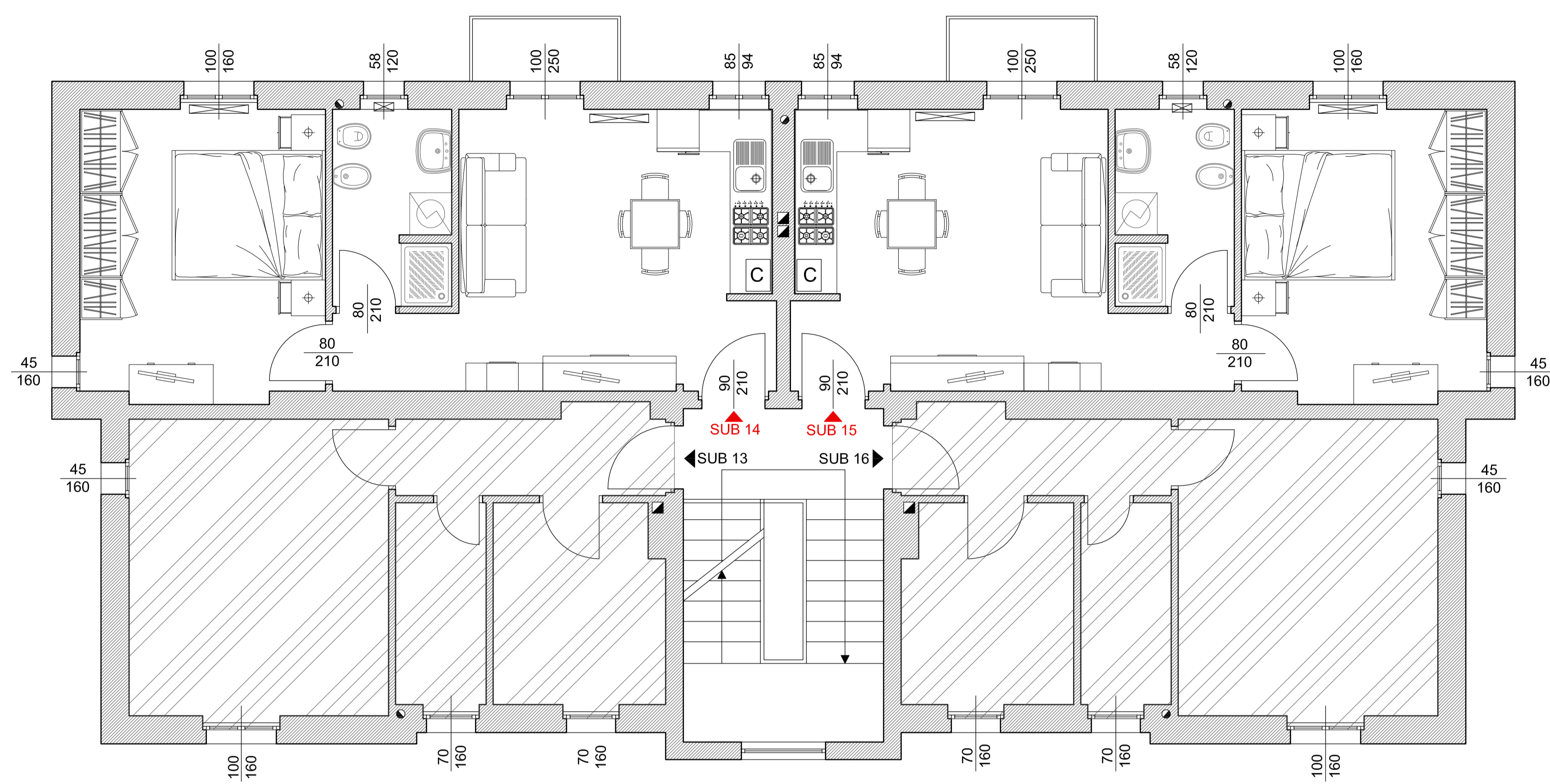
PIANTA QUOTATA - PIANO TERZO - SCALA 1:50
