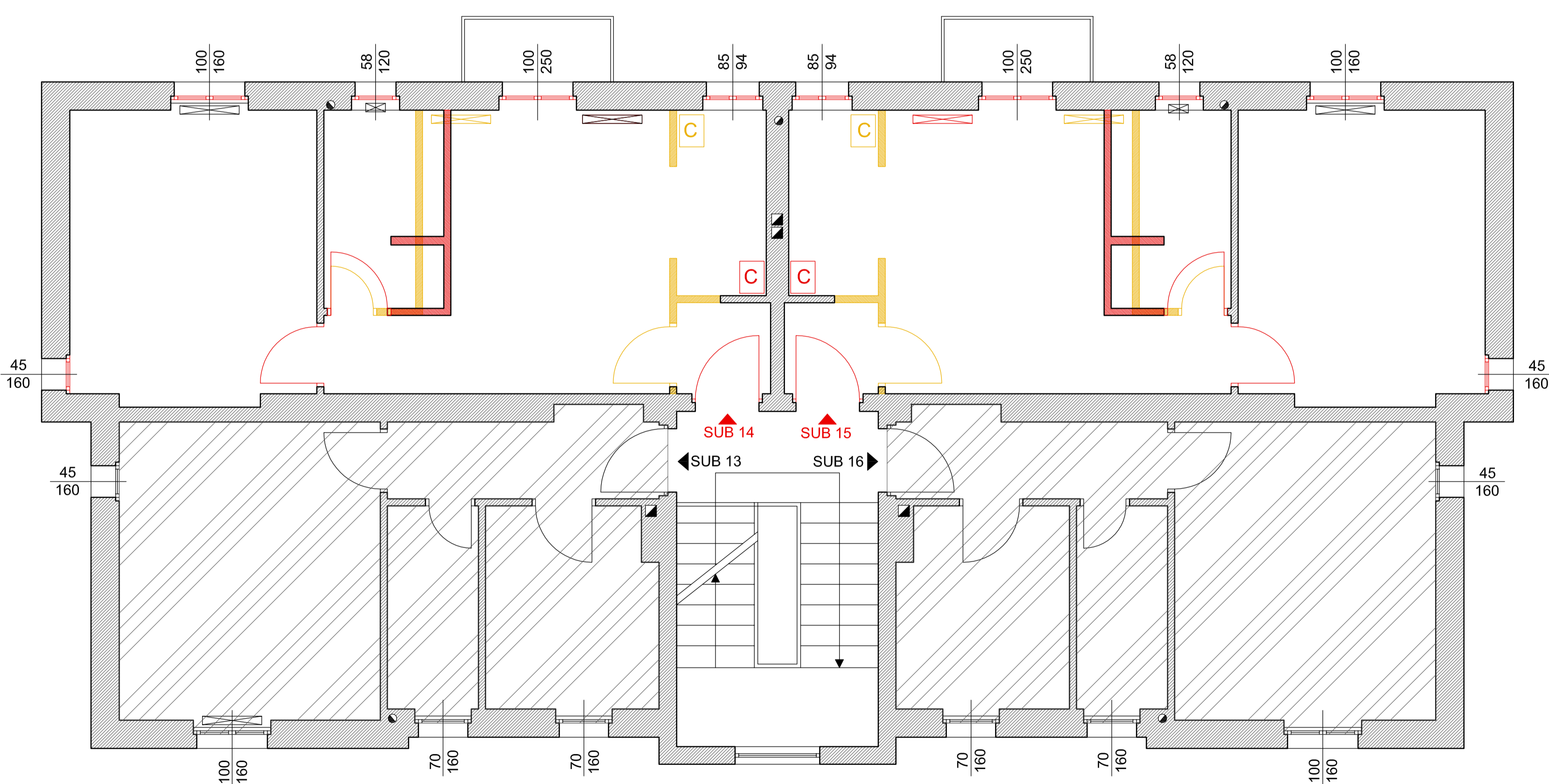
STATO DI CONFRONTO - PIANO TERZO - SCALA 1:50
