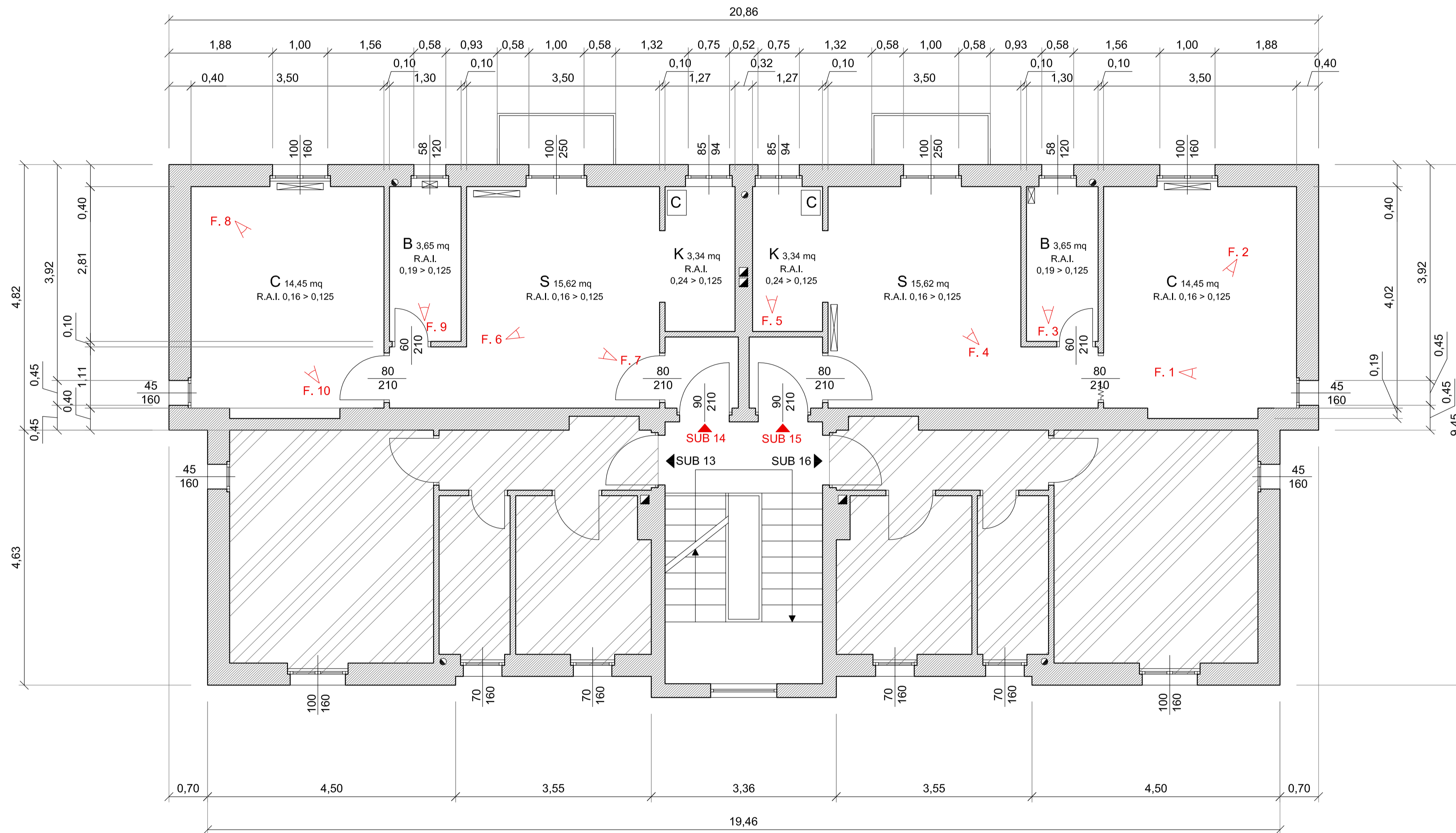
STATO DI FATTO - PIANO TERZO - SCALA 1:50
