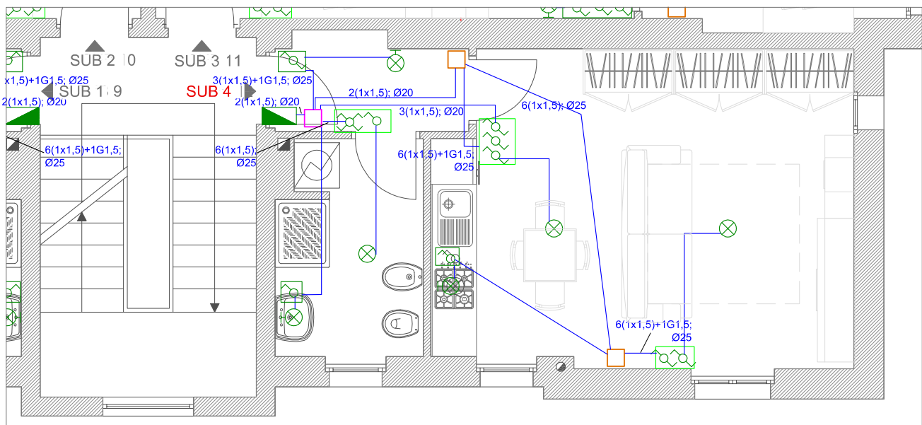
PIANTA IMPIANTO LUCI - VIA VIVAI 3/B, PAVIA - PIANO PRIMO, SUB 4 - SCALA 1:50
